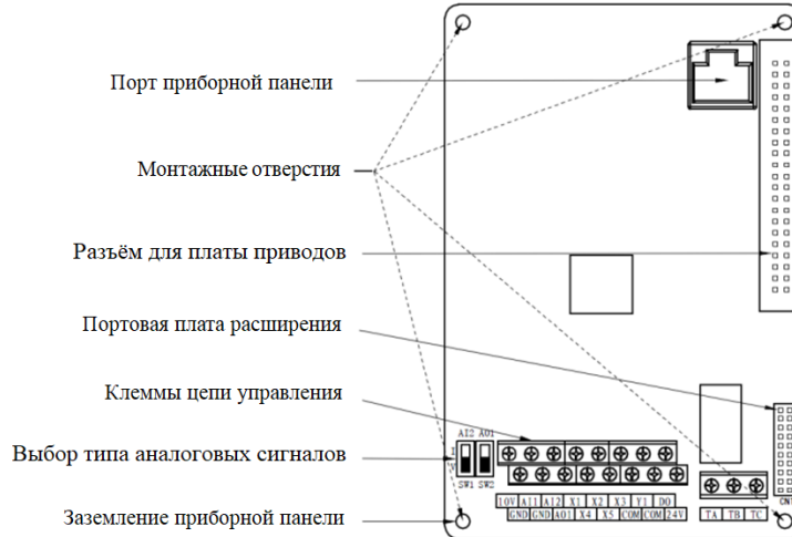
Рис. 3-16 Плата управления
